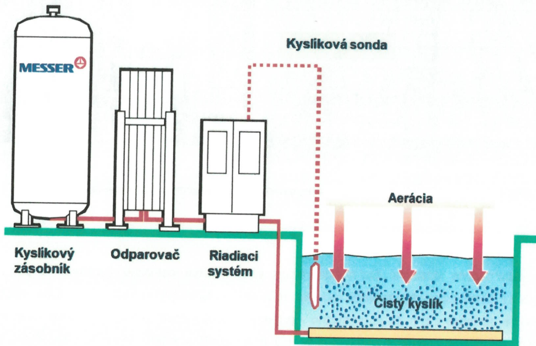
Obr. 1 - Všeobecná schéma dávkovania O 2 cez okysličovacie rošty
