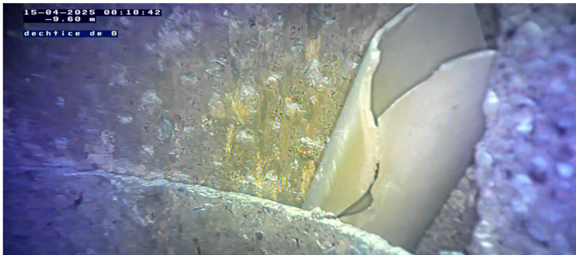
„Zmena priemeru“ a prekážka v hĺbke 9,7 m
